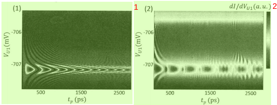
图 3.6 (1) 利用理想方波模拟得到的 Larmor 振荡相图。(2) 在 (1) 图基础上沿垂直方向每条数据点卷积一个高斯函数，模拟噪声影响下的 Larmor 振荡过程。
