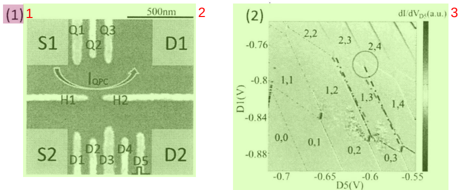
图 4.4 (1) 实验制备的 GaAs 双量子点样品结构图。(2) 利用 QPC 锁相调制技术得到的电荷稳态分布图，我们使量子点工作在图中圆圈标注的 (1-4)-(2,3) 区域。
