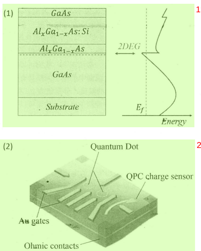
图 1.2 (1) GaAs/AlGaAs 异质结示意图，红色虚线所示为二维电子气 (2DEG) 所在位置。 (2) 门控量子点示意图，灰色结构为纳米加工制作的金属电极。紫色区域为连接 2DEG 的欧姆接触。
