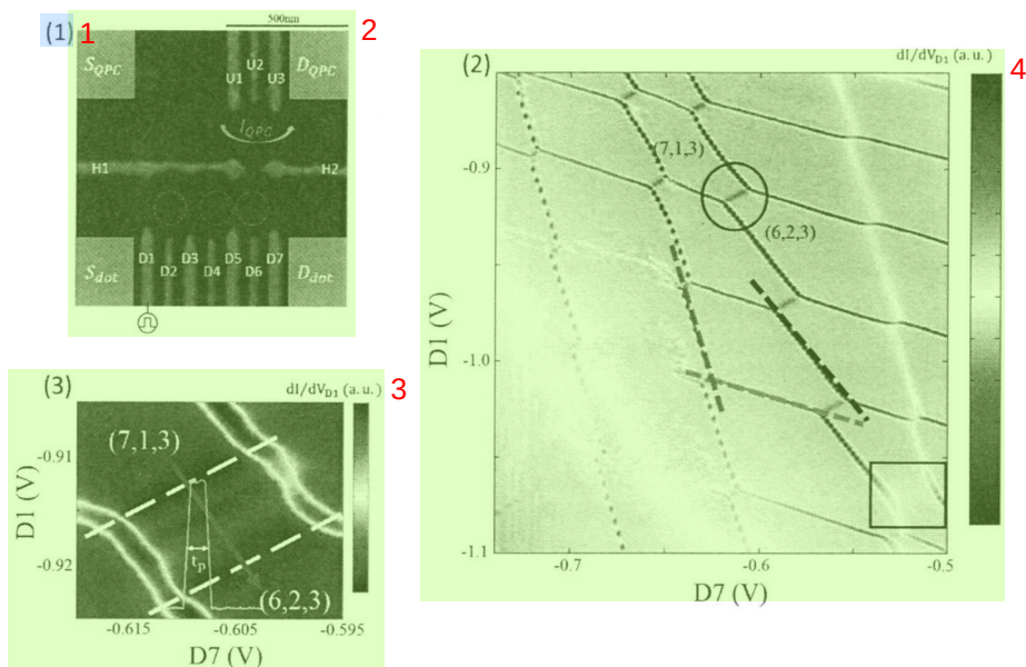
图 6.4 (1) 实验制备的三量子点样品结构图。(2)QPC 锁相调制方法得到的电荷稳态分布图。(3) 施加电压短脉冲后 (7,1,3)-(6,2,3) 区域的隧穿相图。
