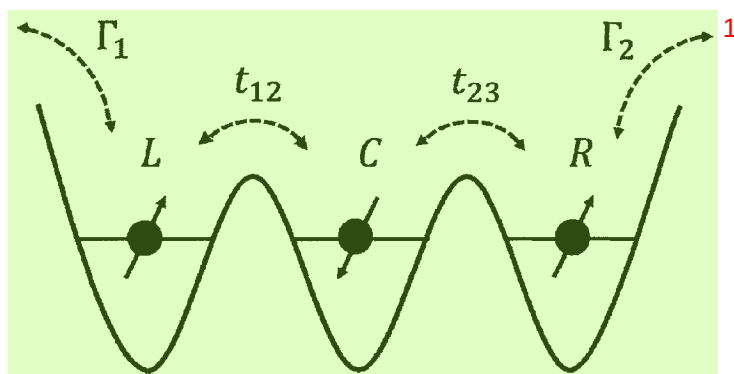
图 6.1 线性耦合三量子点中各占据一个电子。 2
