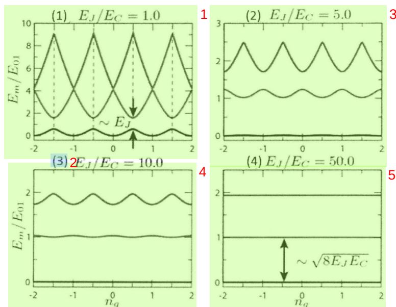
图 4.1 Transmon qubit 能级结构随 E_J/E_C 的变化关系, E_J/E_C 越大, 能级越平行。(图片引自文献 [76])
