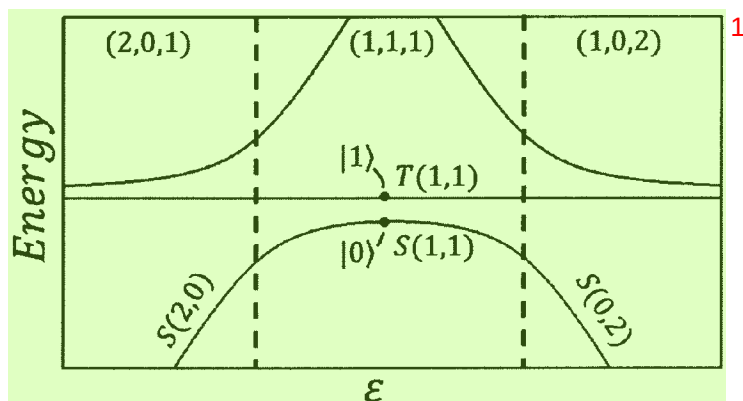
图 6.3 简化后的 exchange qubit 能级结构。
