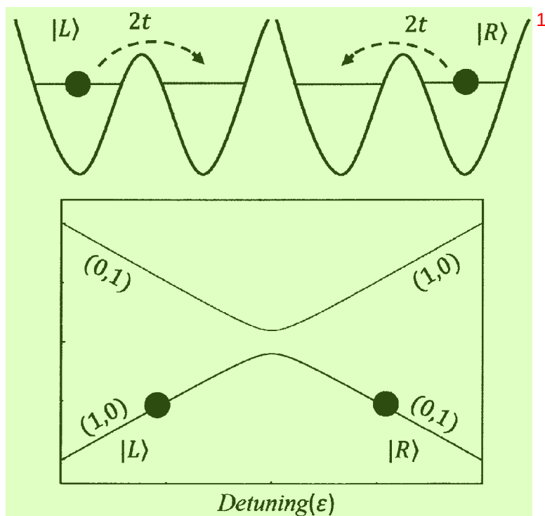
图 3.1 (1)charge qubit 的两个编码状态示意图。(2)两能级体系示意图。 2
