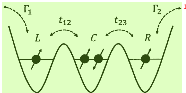
图 5.1 线性耦合的三量子点结构示意图。 2
