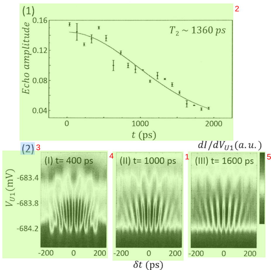
图 3.12 (1) 从实验结果提取的回声幅度随总演化时间 t 的变化关系，从中拟合出非均匀消相干时间 T_2 = 1360 \pm 400 \text{ ps} 。(2) 利用实验数据模拟得到的回声过程。
