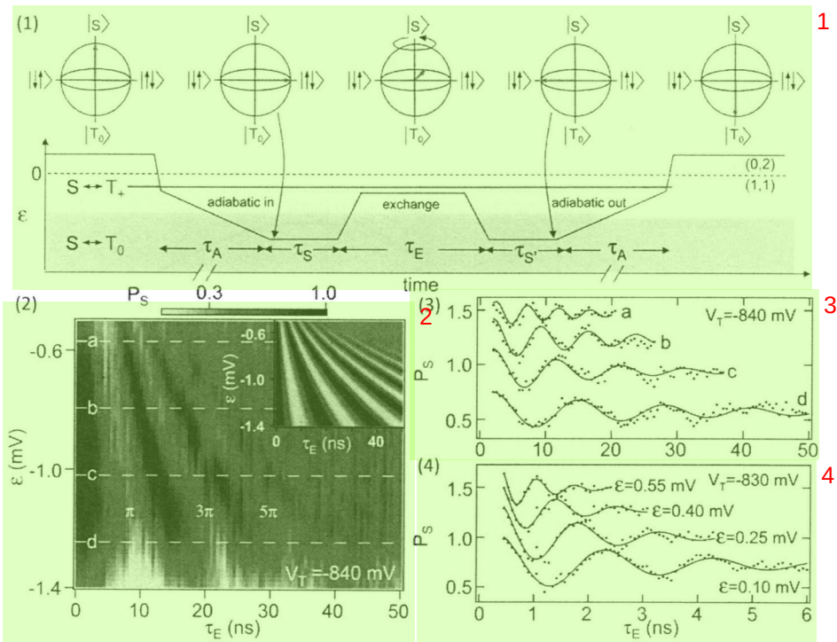
图 2.5 (1) 实现比特交换相互作用驱动下的相干振荡所用脉冲序列示意图。(2) 实验测量得到的 QPC 微分电导信号随失谐量 \epsilon 和演化时间 \tau_E 变化关系，图中可以清晰地分辨出三个相干振荡峰。(3) 从图 (2) 中不同失谐量 \epsilon 处得到的 Rabi 振荡曲线，实线为根据数据拟合得到的结果。(4) 增加双点间隧穿耦合强度 2t 后得到的更快速的 Rabi 振荡过程。（图片引自文献 [32]）
