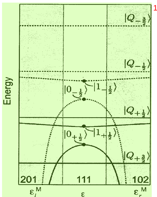
图 6.2 Exchange-only qubit 能级结构图。(图片引自文献 [87])
