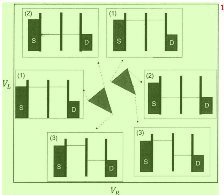
图 1.7 双量子点输运测量结果。(1) \mu_L = \mu_R = \mu_S 。(2) \mu_L = \mu_R = \mu_D 。(3) \mu_L = \mu_S 及 \mu_R = \mu_D (图片引自 Ke Wang PhD Thesis)。
