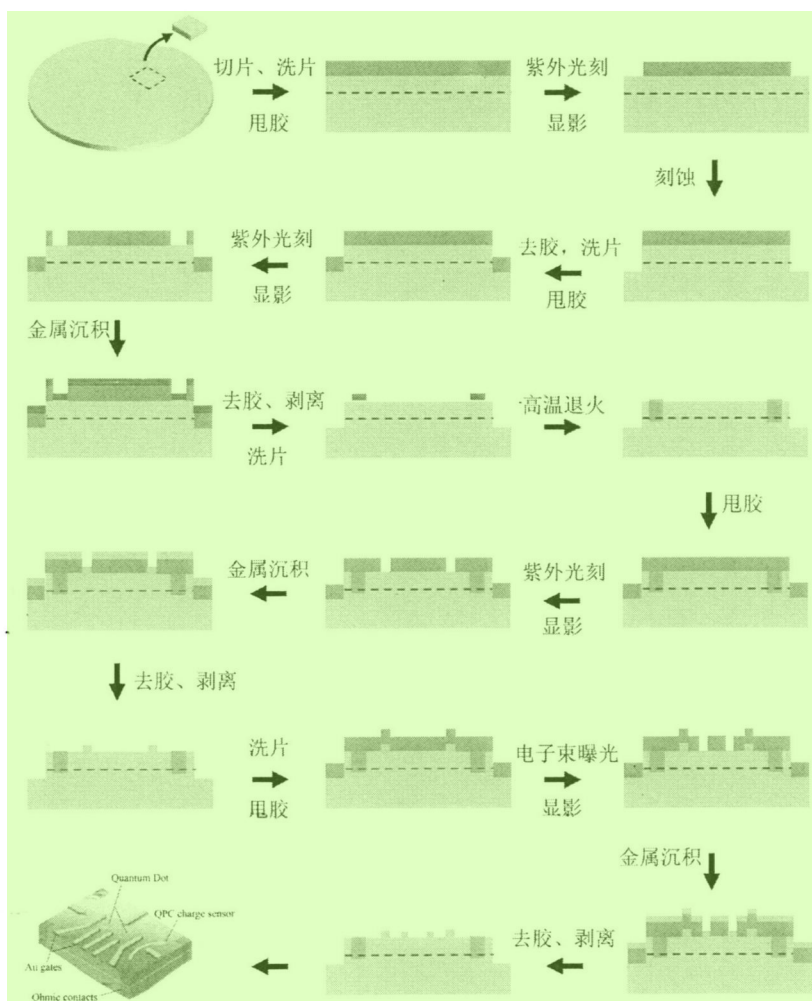
图 1.9 掺杂 GaAs/AlGaAs 异质结量子点制备工艺流程图。浅蓝色区域为半导体材料基片，绿色为紫外光或电子抗蚀剂，棕色为欧姆接触金属，黄色为表面栅电极金属。
