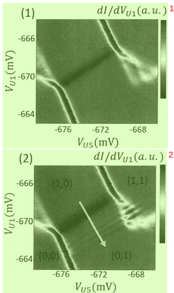
图 3.3 (1) 图 3.2.2 中红色圆圈所示的双点反交叉区域。(2) 通过在电极 U1 上施加电压短脉冲，重复扫描 (1) 图得到。
