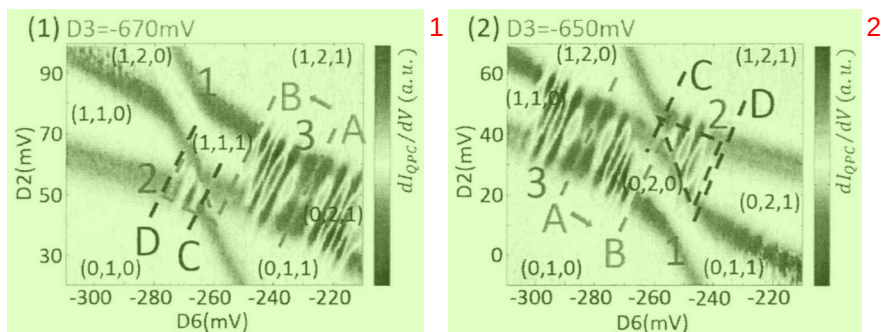
图 5.4 (1) 在电极 D1 施加 15GHz 的微波信号后得到的电荷稳态分布图。(2) 通过调节电极 D4 使三量子点电化学势相互高度发生位移，重复 (1) 中过程得到的结果。
