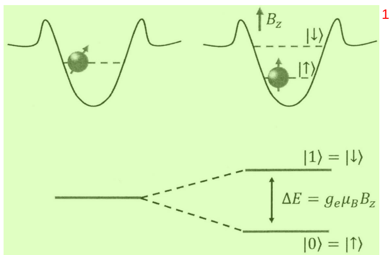
图 2.1 单电子自旋态示意图
