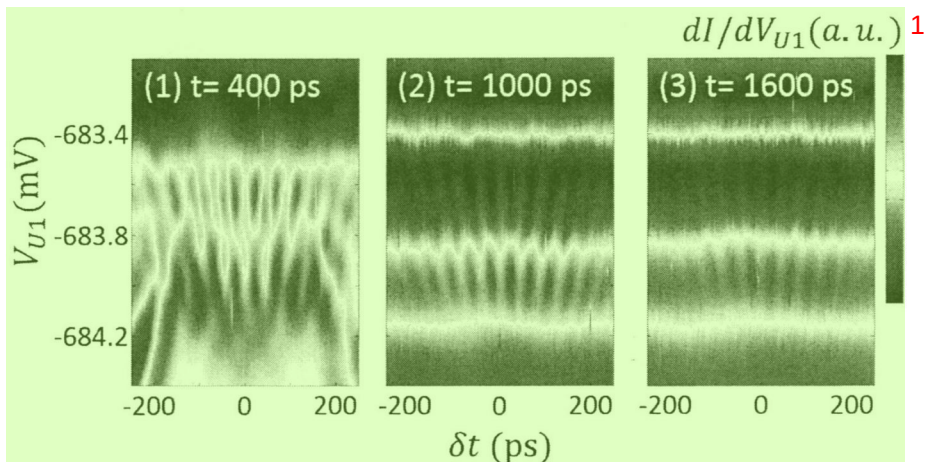
图 3.11 测量得到的 QPC 微分电导随电压 V_{U1} 和演化时间 \delta t 的变化关系，(1)、(2) 和 (3) 分别对应总演化时间 400、1000 和 1600ps。
