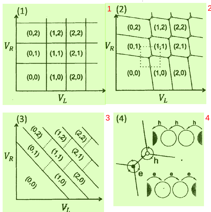
图 1.6 双量子点相图。(1) 两个量子点间没有耦合，为两个孤立的单点。(2) 量子点间存在隧穿耦合，但耦合较弱。(3) 量子点间耦合非常强，逐渐融合成一个大的单量子点。(4) 三相点示意图。e 和 h 分别表示电子和空穴输运过程。(图片引自文献 [29])
