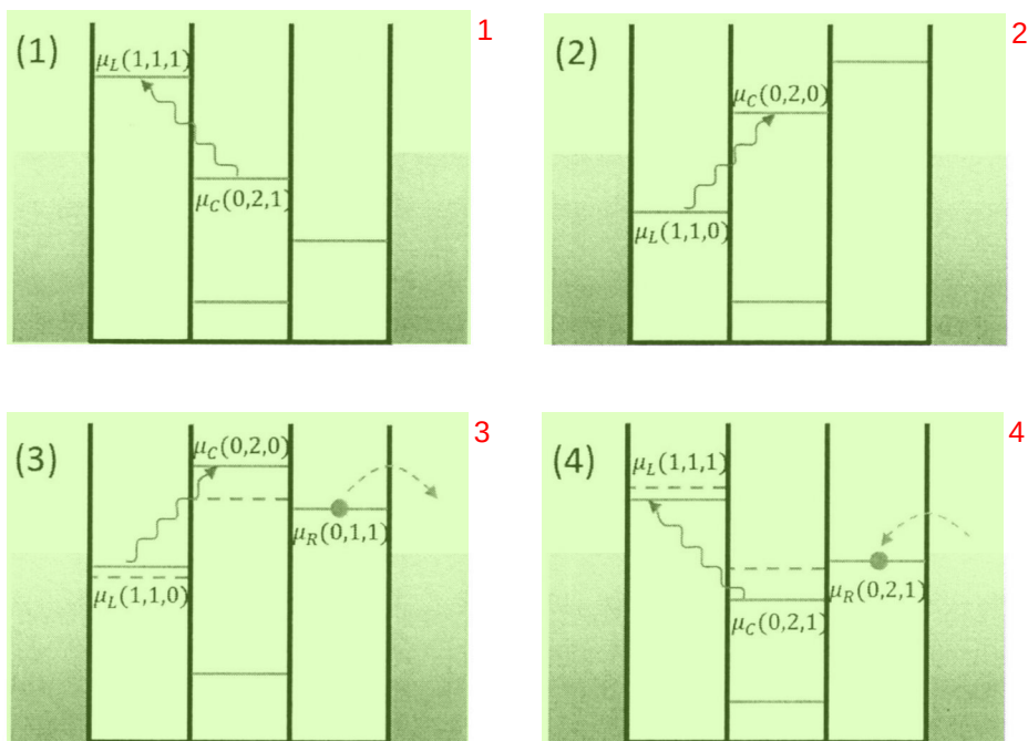
图 5.5 (1) 图 5.4.1 区域 3 中 PAT 过程示意图。(2) 图 5.4.2 区域 3 中的 PAT 过程示意图。(3) 图 5.4.1 区域 2 中 PAT 过程示意图。(4) 图 5.4.2 区域 2 中 PAT 过程示意图。
