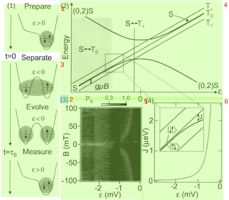
图 2.4 (1) 对双量子点 S - T_0 态进行操控时电子态变化示意图。(2) 在外加磁场作用 B_z 下 (1,1)-(0,2) 反交叉区域能级示意图。(3) 实验测量得到的 S - T_+ 交叉点所在位置随外磁场变化关系。(4) S - T_0 交换相互作用 J 的大小随失谐量 \epsilon 的变化关系。(图片引自文献 [32])
