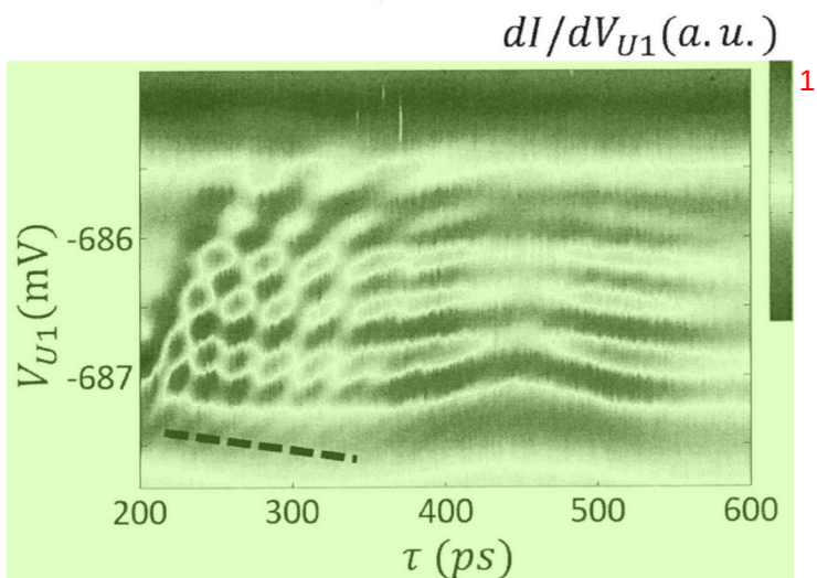
图 3.8 实验中测得的 QPC 微分电导随电压 V_{U1} 和自由演化时间 t_p 的关系。
