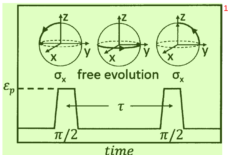
图 3.7 实现 Ramsey 干涉实验的非绝热脉冲示意图及比特状态在 Bloch 球上的演化过程。
