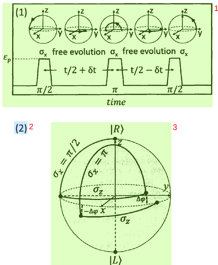
图 3.10 (1)charge echo 所采用的非绝热脉冲示意图以及对应的比特状态在 Bloch 球上演化过程。(2)echo 翻转消除噪声扰动的一种直观理解, 两次 \sigma_z 转动过程中产生的轨迹偏移量 \Delta\phi 相互抵消。
